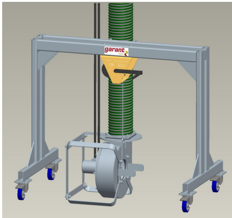
Bild 1: Power-Filling-Aid mit Saugschlauch NW 150 und mobiler Hub- und Senkvorrichtung.
